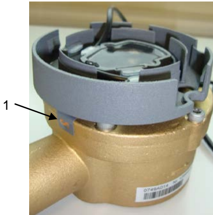
Im Werk angebrachte Plombierungen am Durchflusssensor (1) und am Temperaturfühler (2) des Superstatic 749
