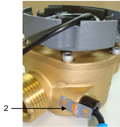
Im Werk angebrachte Plombierungen am Durchflusssensor (1) und am Temperaturfühler (2) des Superstatic 749
