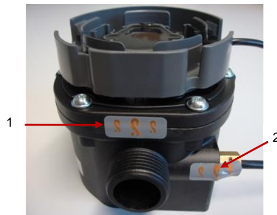
Sigilli di fabbrica sulla volumetrica (1) e sulla sonda di temperatura (2) del Superstatic 789
