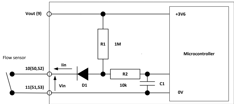
Schéma électrique mode normal
